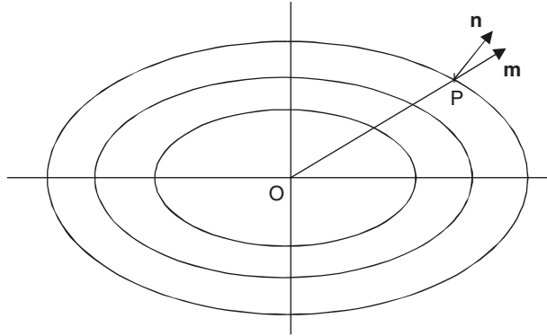
Figure 9.28 Equipotential ellipses.
